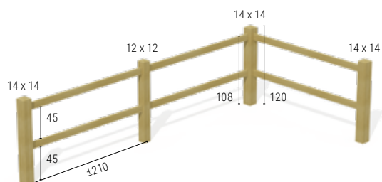
Type 1 met 2 horizontale liggers
