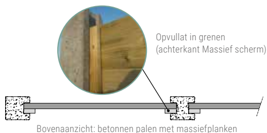
Massief scherm okan in betonnen gleufpalen met plaat onderaan
