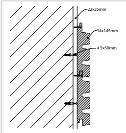
geïmpregneerd grenen of thermo-ayous 35 x 145 mm
