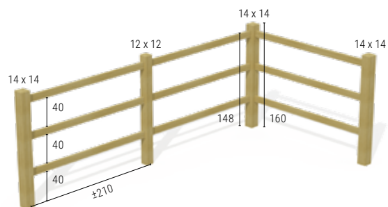
Type 2 met 3 horizontale liggers
