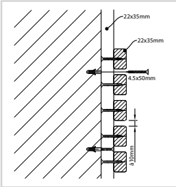
padouk 22 x 35 mm
