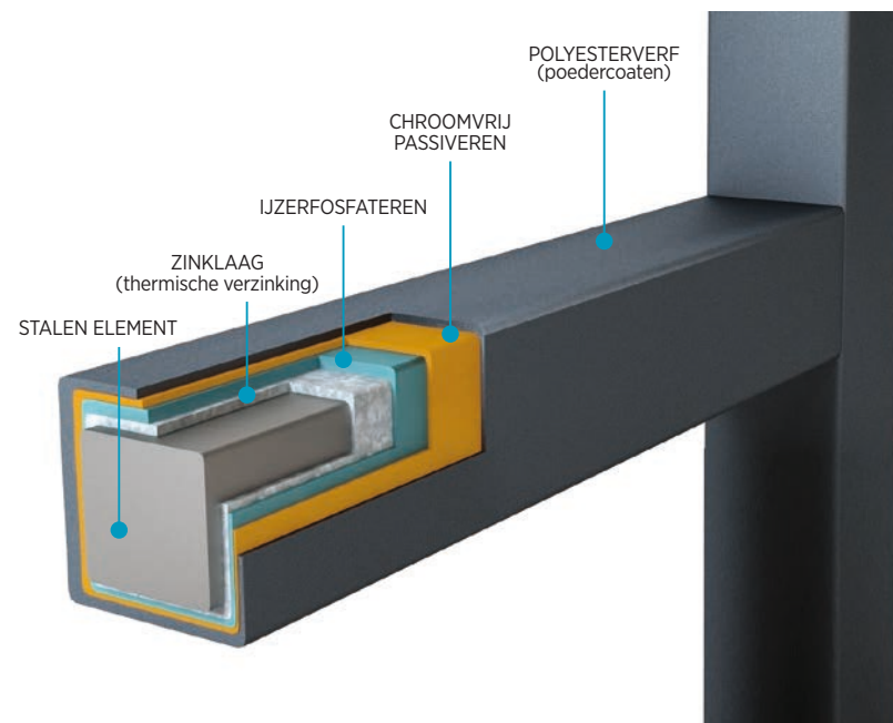
Doorsnede van het element beveiligd in het DUPLEX systeem.
