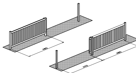
Op rails
