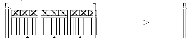
Schuifpoort decoratief (hoogte: 180 cm)
