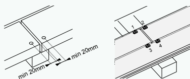
Aansluitende plaatsing op een draagbalk
