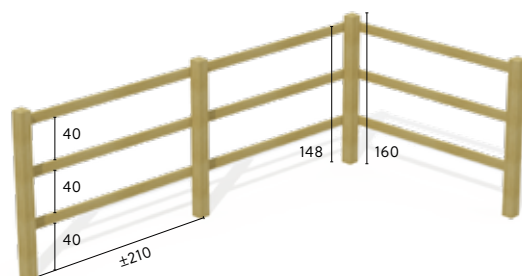
Type 2 met 3 horizontale liggers
