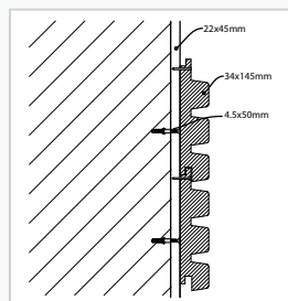
geïmpregneerd grenen, padouk of thermo-ayous 35 x 145 mm TRIPLE
